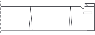
PROFILO DI FINITURA PERIMETRALE PER POSA FLOTTANTE PERIMETER PROFILE FOR FREE-FLOATING INSTALLATION
