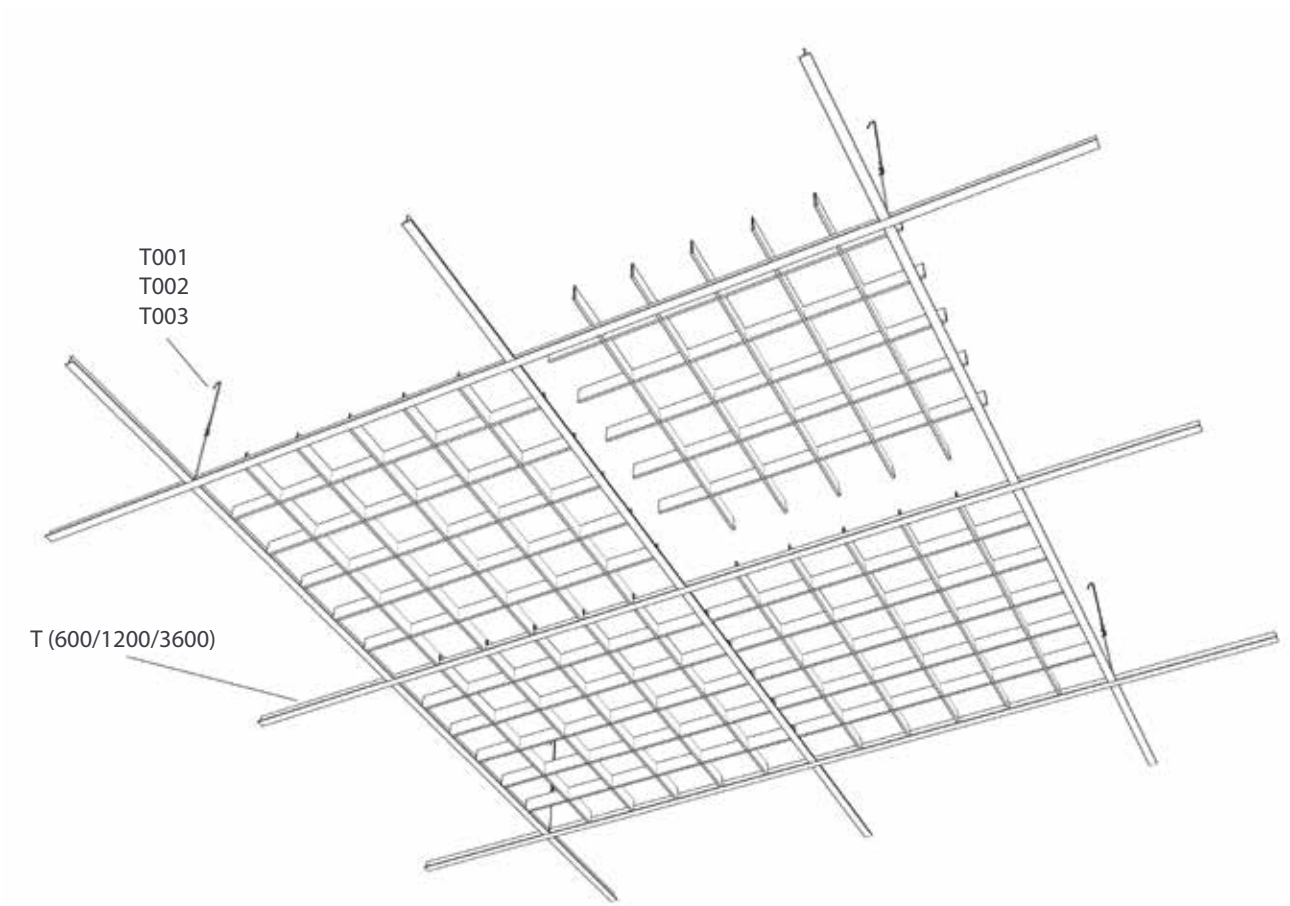
SISTEMA DI MONTAGGIO A FILO TO LAY-ON SYSTEM
